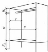
图 5-75 衣柜尺寸标注
